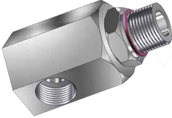
RADYAL (90°) BAĞLANTILI
